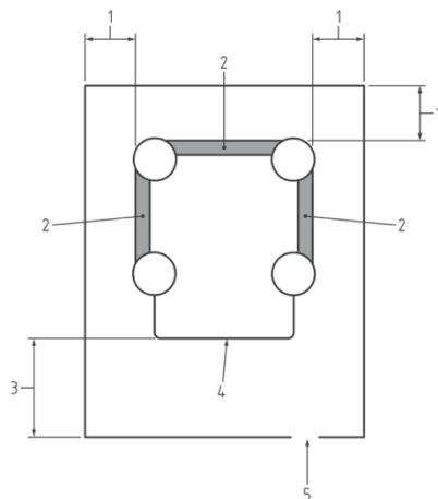
Figuur 2 EN 14960 Plaatsing
