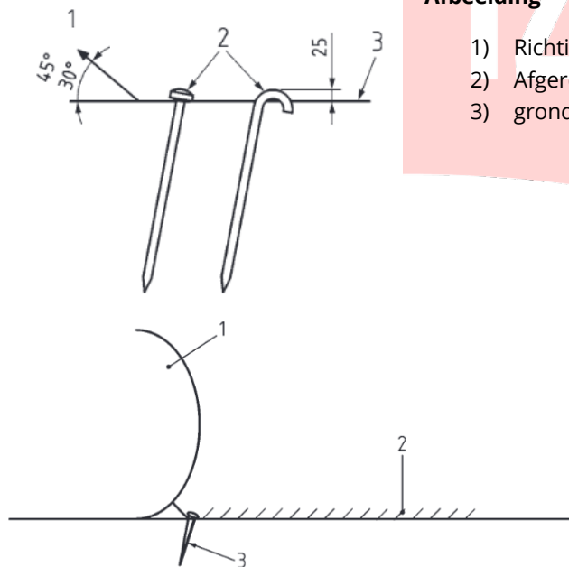
Figuur 6 EN 14960 Impactzone
